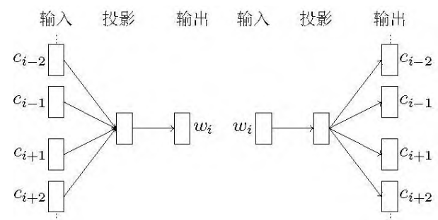
图 3 CBOW 与 SG 框架图
