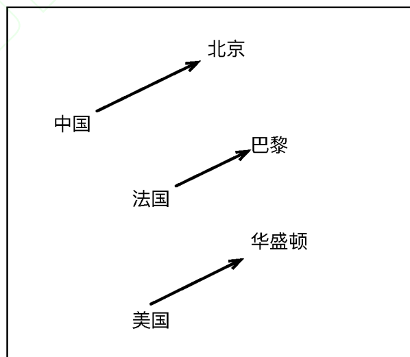
图 5 单词类比示意图(利用 PCA 将单词向量表示降维到 2 维后示意图，途中箭头所示为使用对应的首都的向量减去国家向量表示后得到的向量)
