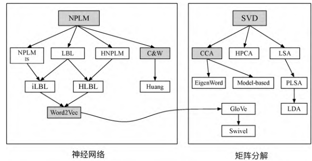
图1 单词表示学习代表性方法发展示意图,方框节点为代表性模型,箭头所示为模型影响方向,加灰节点为本节重点介绍模型,因其衍生出大量后续工作。注意,此图中只列出了代表性工作,省略了大量的细节工作,如C&W、Word2Vec、CCA等,都有大量衍生工作。
