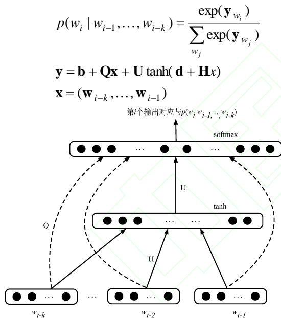
图 2 神经网络语言模型
